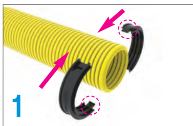
RKSC: assemblaggio
